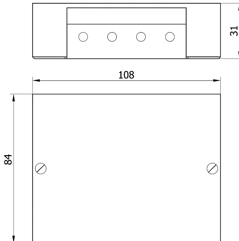
Рисунок 1 - Габаритный чертеж корпуса
